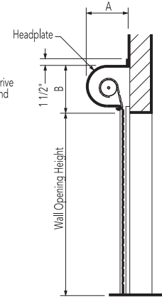
Section A-A
